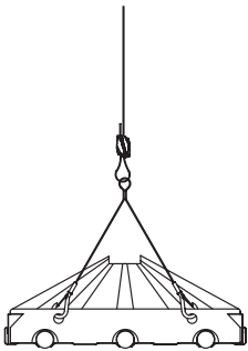
Akcesorium Y-Fit z haczykiem zatraskowym z oprawą oświetleniową
