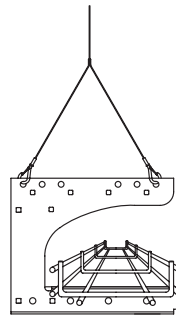
Y-Fit z haczykiem zatraskowym na wsporniku G - mocowanie koryta
