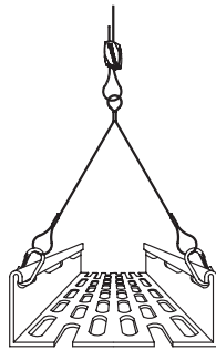
Akcesorium Y-Fit z karabińczykiem - mocowanie koryta kablowego
